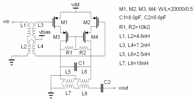
Fig. 6. The 29 dBm optional PA schematic
